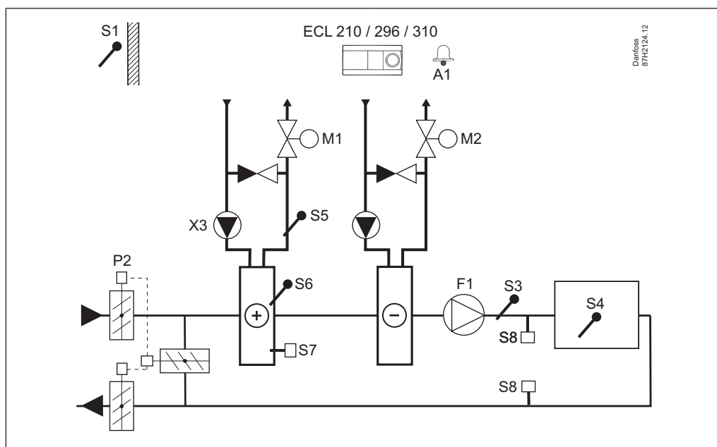
A214.5, przykład a: Aplikacja grzewcza/chłodnicza, temperatura w kanale oparta na temperaturze w pomieszczeniu
