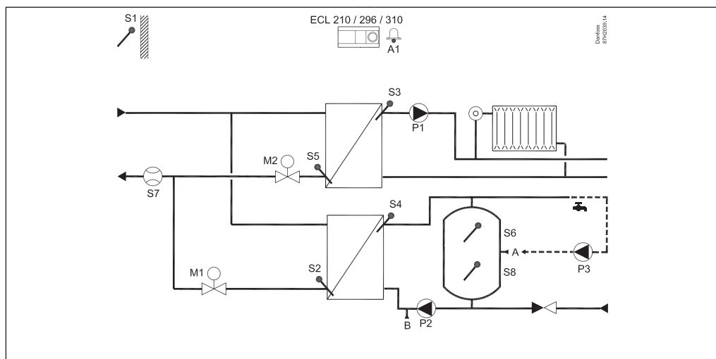
A247.1, przykład a: Układ ogrzewania i ładowania zasobnika CWU podłączony pośrednio. Praca równoległa lub priorytet CWU
