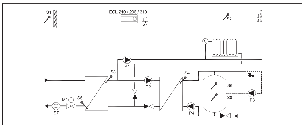
A247.1, przykład a: Układ ogrzewania i ładowania zasobnika CWU podłączony pośrednio. Praca równoległa lub priorytet CWU
